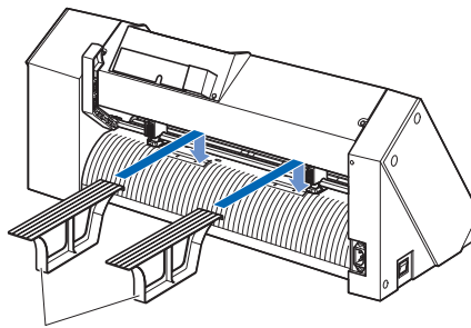
Mesa de hoja portadora
